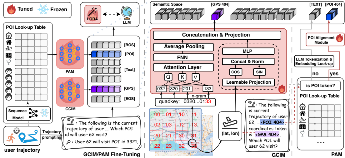
图 3-1 大小模型协同框架示意，图中重点展示 GA-LLM 主推理链路，以及 GCIM 与 PAM 在输入侧的注入流程；其中 PAM 用于承接结构侧（含小模型）学习到的兴趣点关系信息并映射到大语言模型语义空间，最终前 K 个由 GA-LLM 单路输出。
