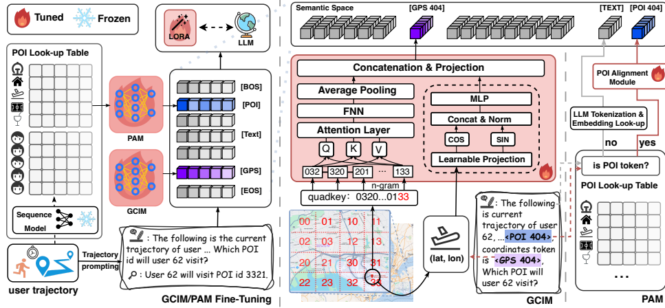
图 3-1 大小模型协同框架示意，图中重点展示 GA-LLM 主推理链路，以及 GCIM 与 PAM 在输入侧的注入流程；其中 PAM 用于承接结构侧（含小模型）学习到的兴趣点关系信息并映射到大语言模型语义空间，最终前 K 个由 GA-LLM 单路输出。
