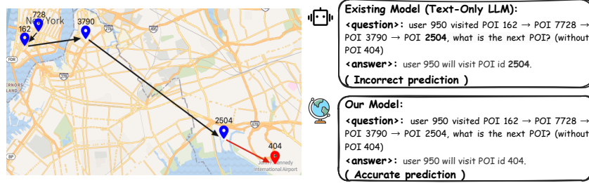
图 1-2 转移先验注入挑战示意，仅依赖词元语义难以恢复兴趣点图中的高阶迁移关系。
