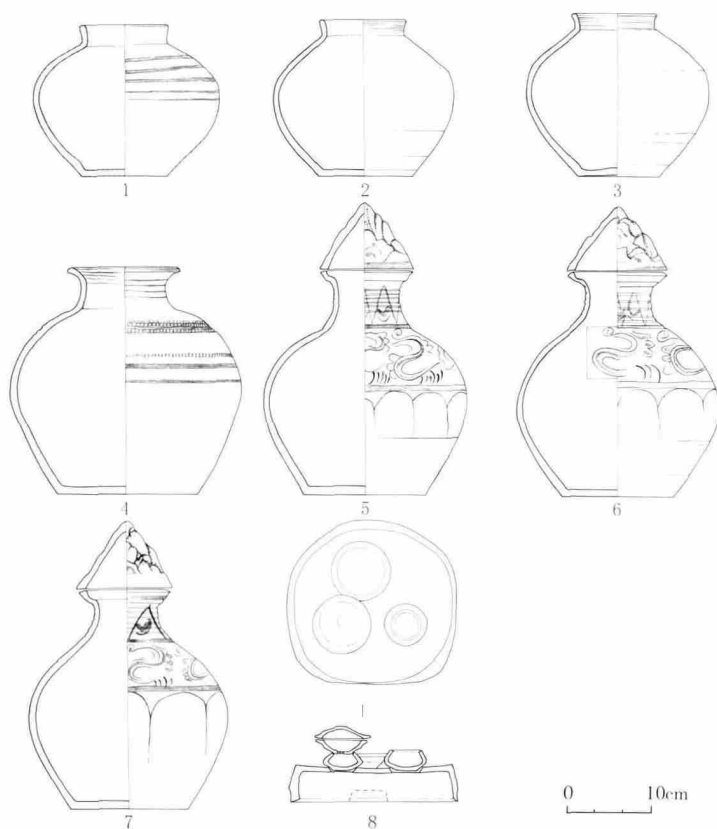
图一九 M101 随葬器物
