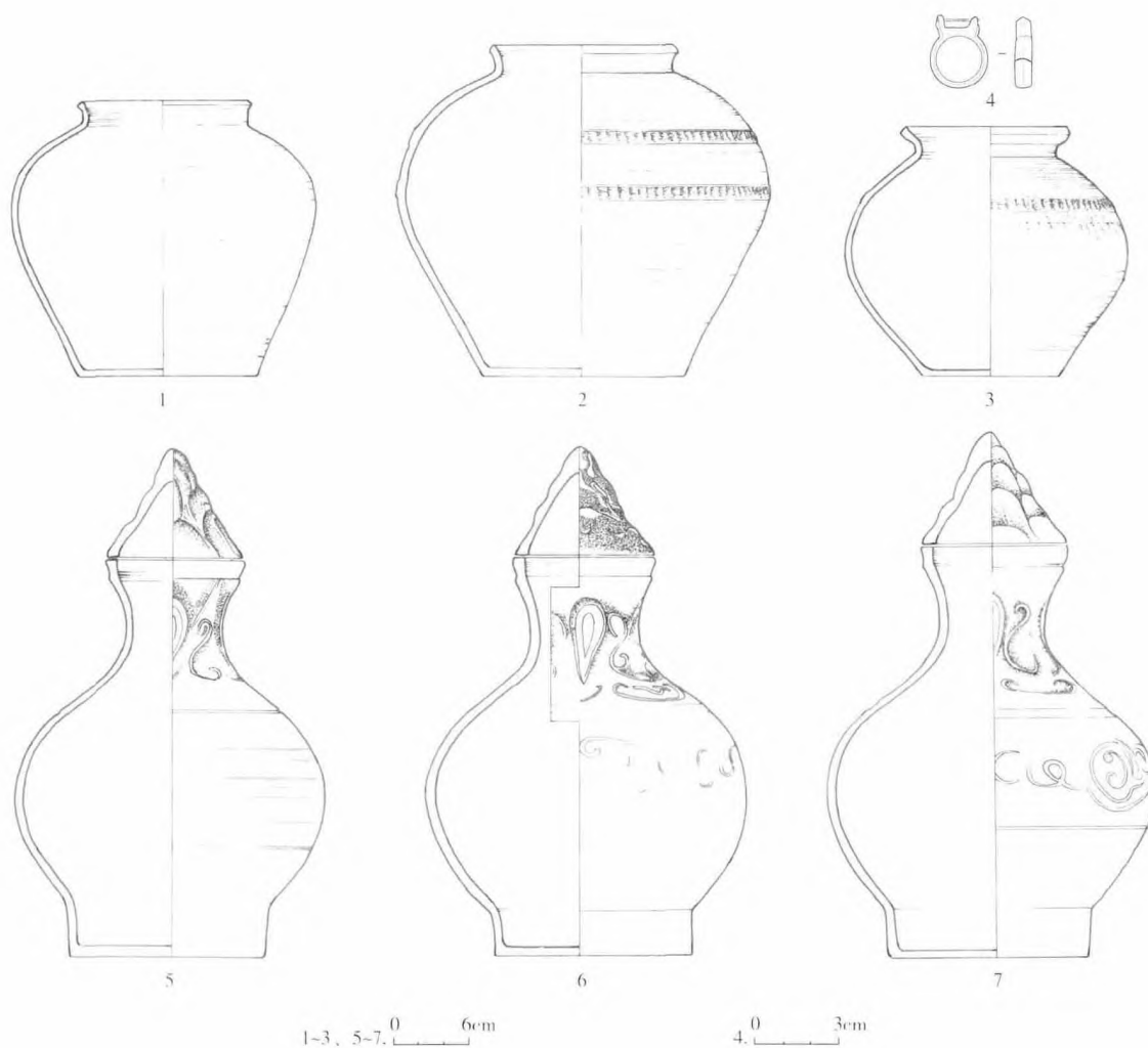
图一一 M5 随葬器物
