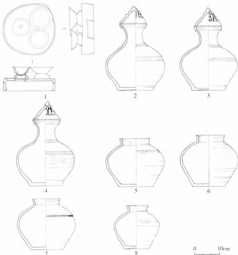
图一七 M66 随葬器物
