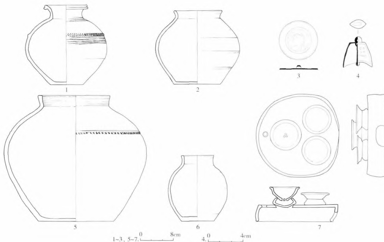
图二三 M17 随葬器物
