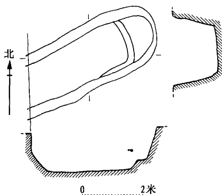
图四 H15 平、剖面图
