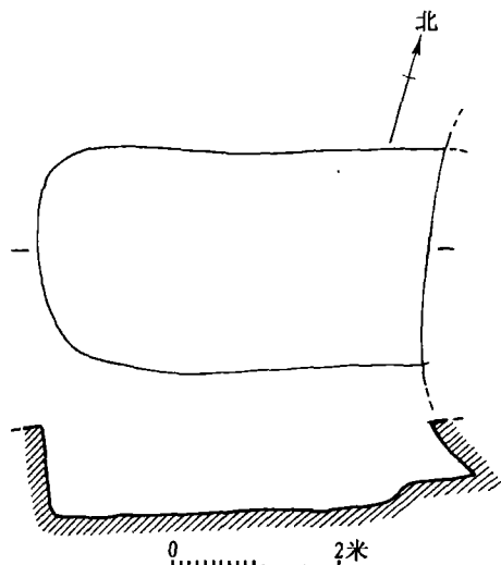
图三 H13 平、剖面图
