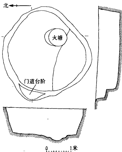
图六 F3平、剖面图
