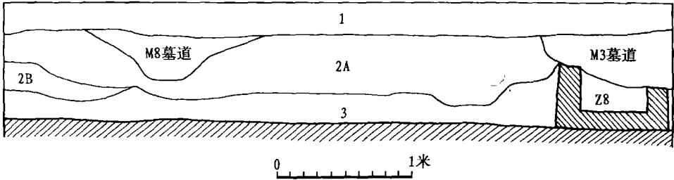
图二 T1001 南壁地层剖面图 1. 耕土层 2A. 灰土层 2B. 灰土和烧土混杂层 3. 褐色土层
