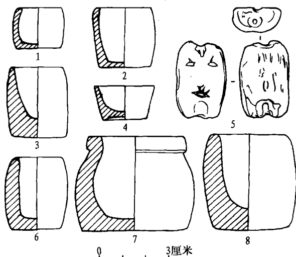
图一七 出土陶器
