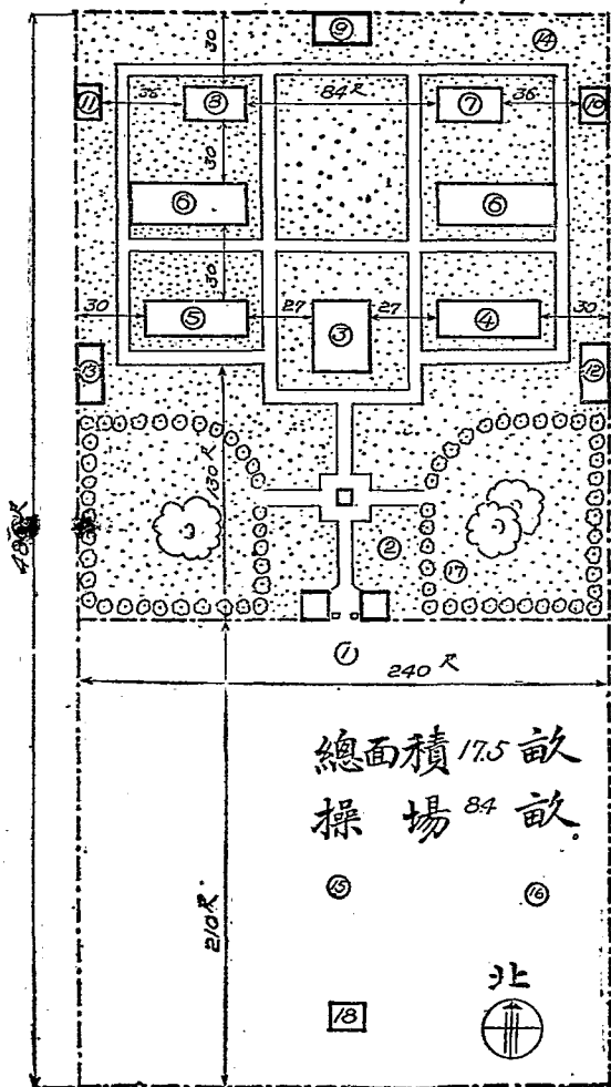
保國民學校校舍標準地盤圖
