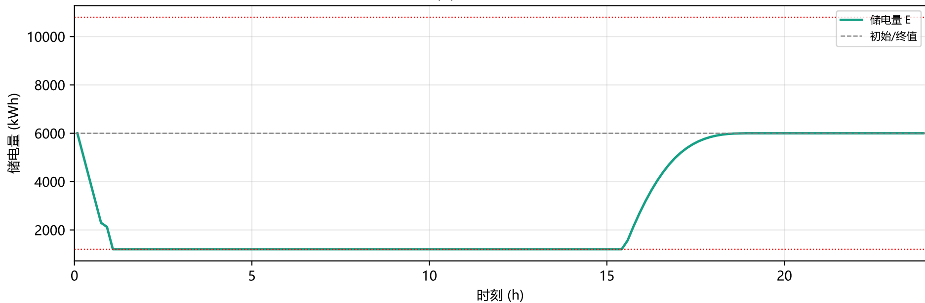
(b) 储能 SOC 轨迹
