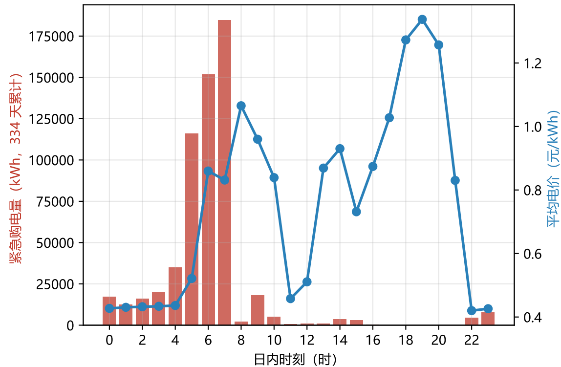
(a) 紧急购电集中于清晨 5-7 时 (光伏预报偏乐观)
