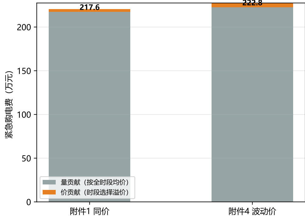
(b) 紧急购电费的数量×价分解
