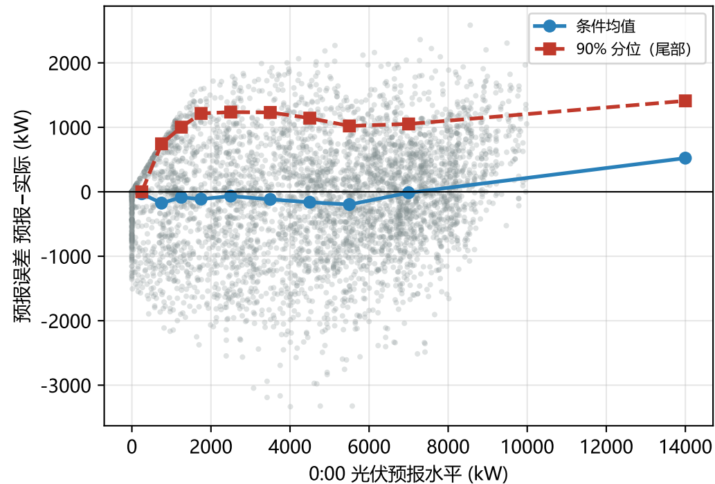
(a) 误差 vs 预报水平 (异方差, 尾部随预报增大)
