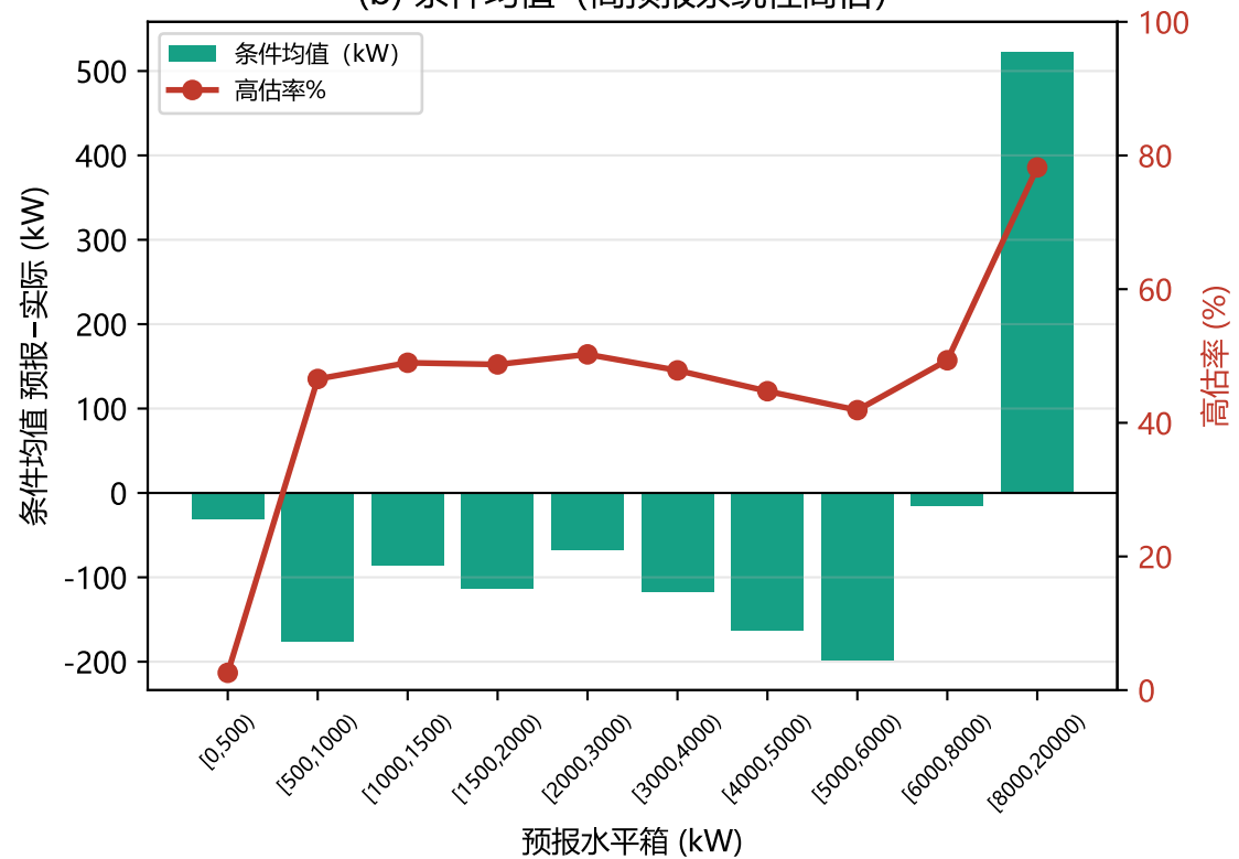
(b) 条件均值 (高预报系统性高估)
