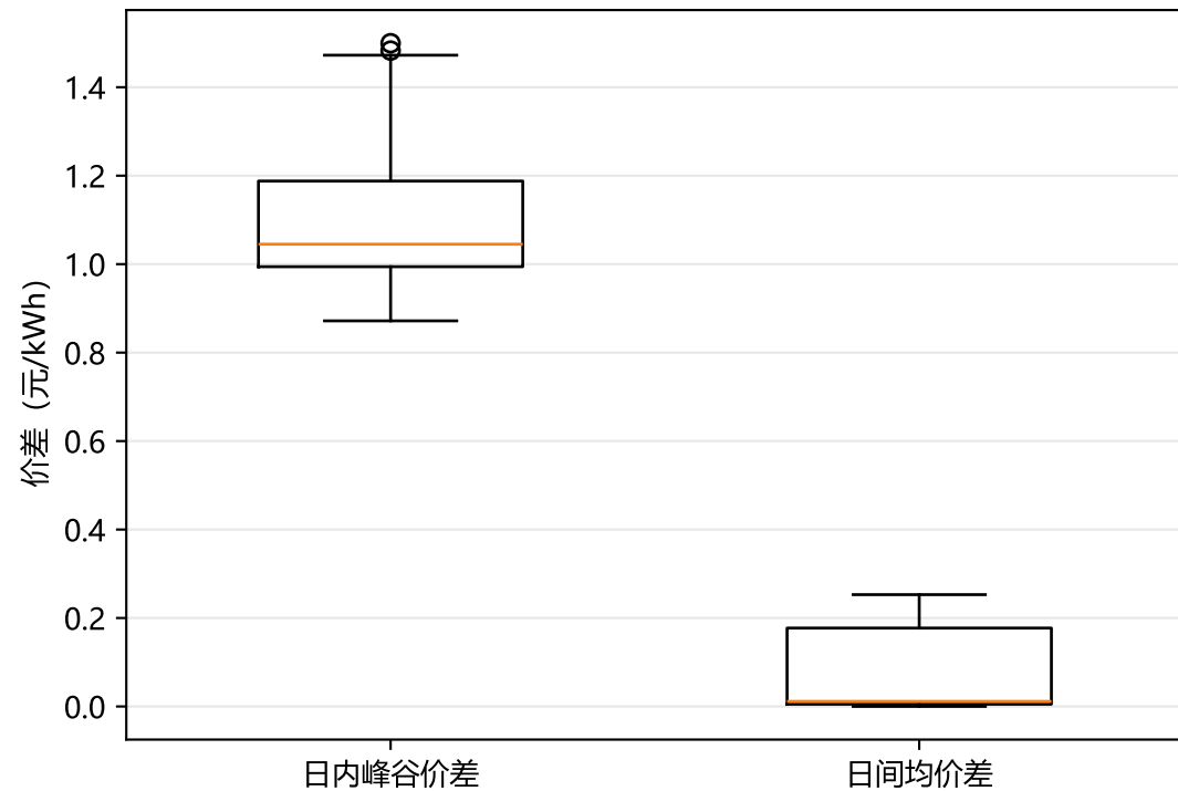
(a) 附件4：日内价差远大于日间价差
