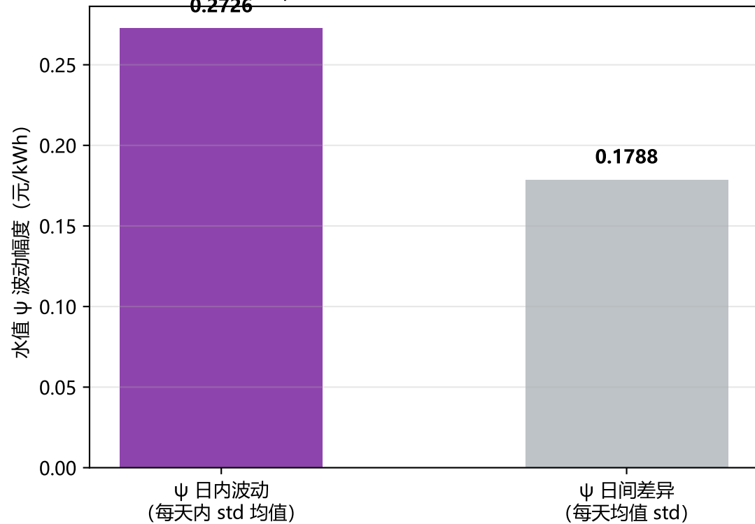
(b) 水值 \psi 几乎全来自日内 (跨日套利空间小)
