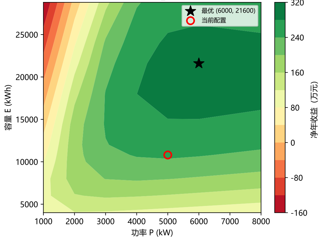
(b) 净年收益 NB(E,P) ( c_E=1000 元/kWh)
