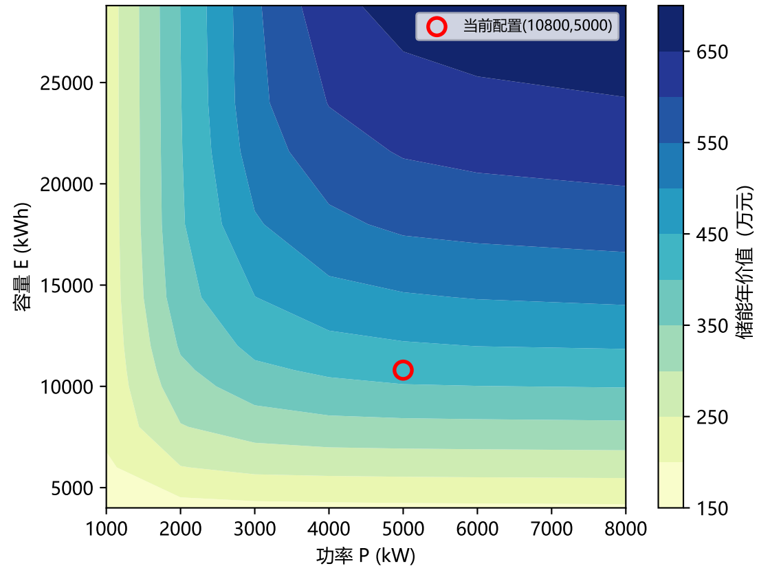
(a) 储能年价值 V(E,P)
