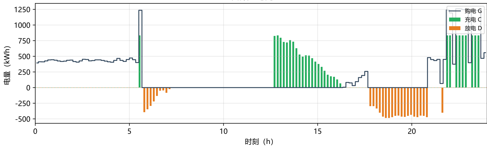
充放电与购电量
