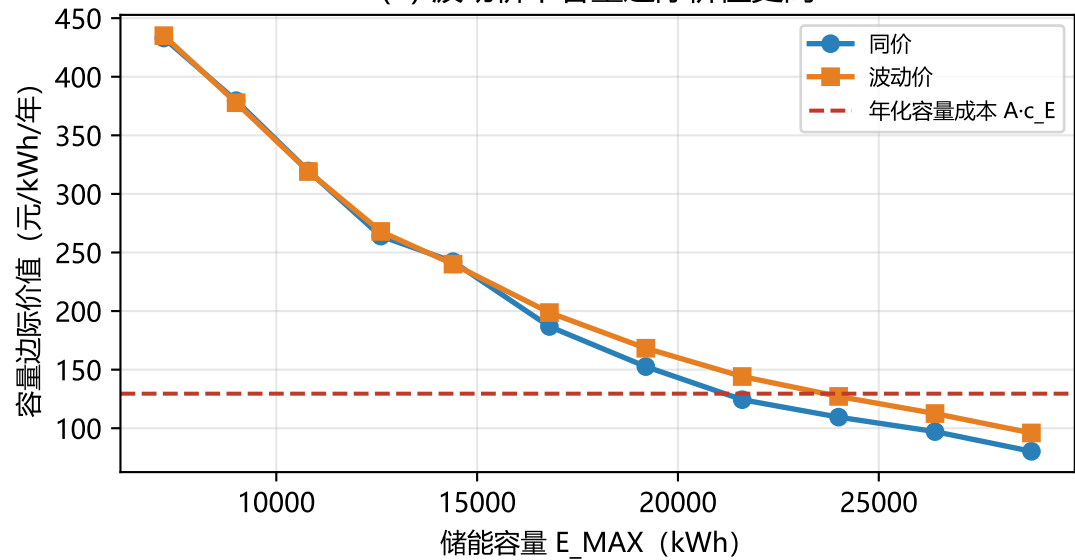
(b) 波动价下容量边际价值更高
