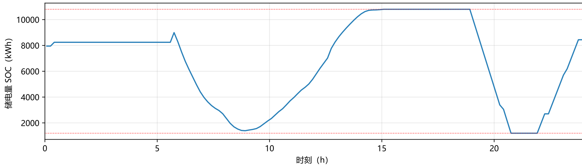
储电量轨迹 (低影子价充电、高影子价放电)
