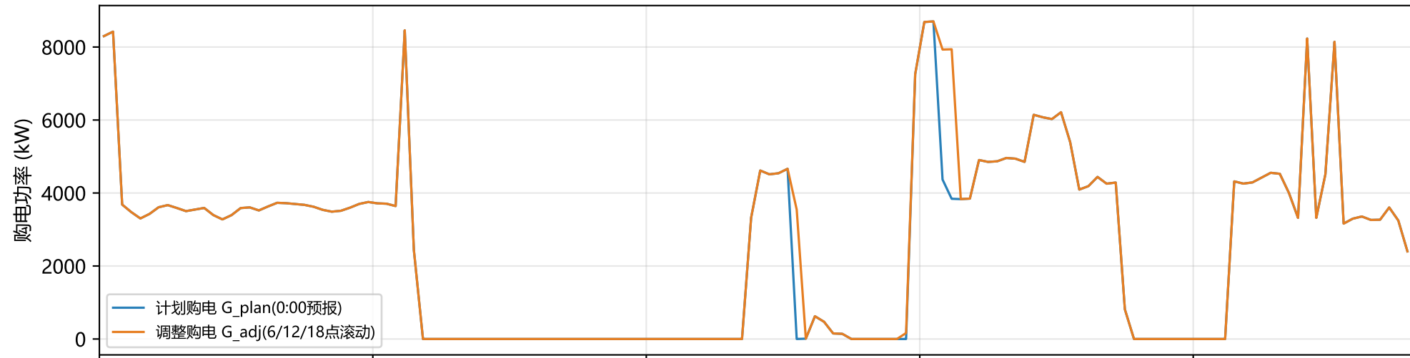
上调量与紧急购电
