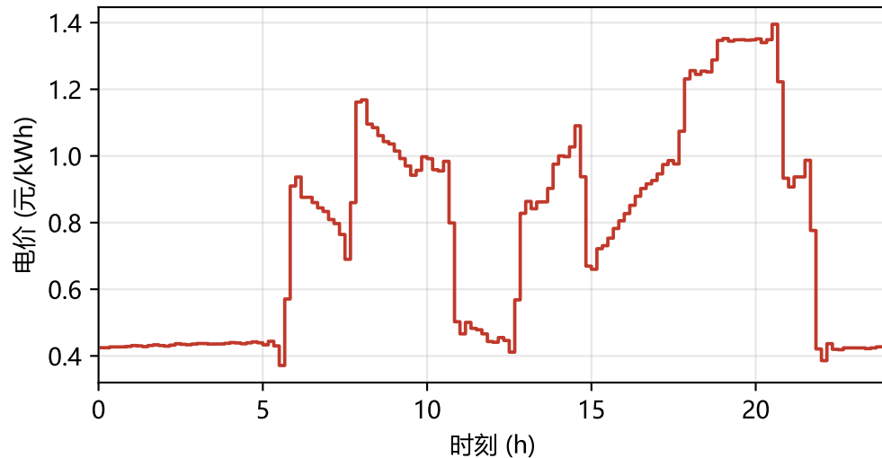
(a) 分时电价
