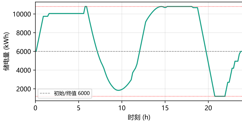
(d) 储能 SOC
