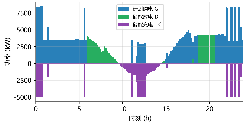
(c) 购电与储能充放电
