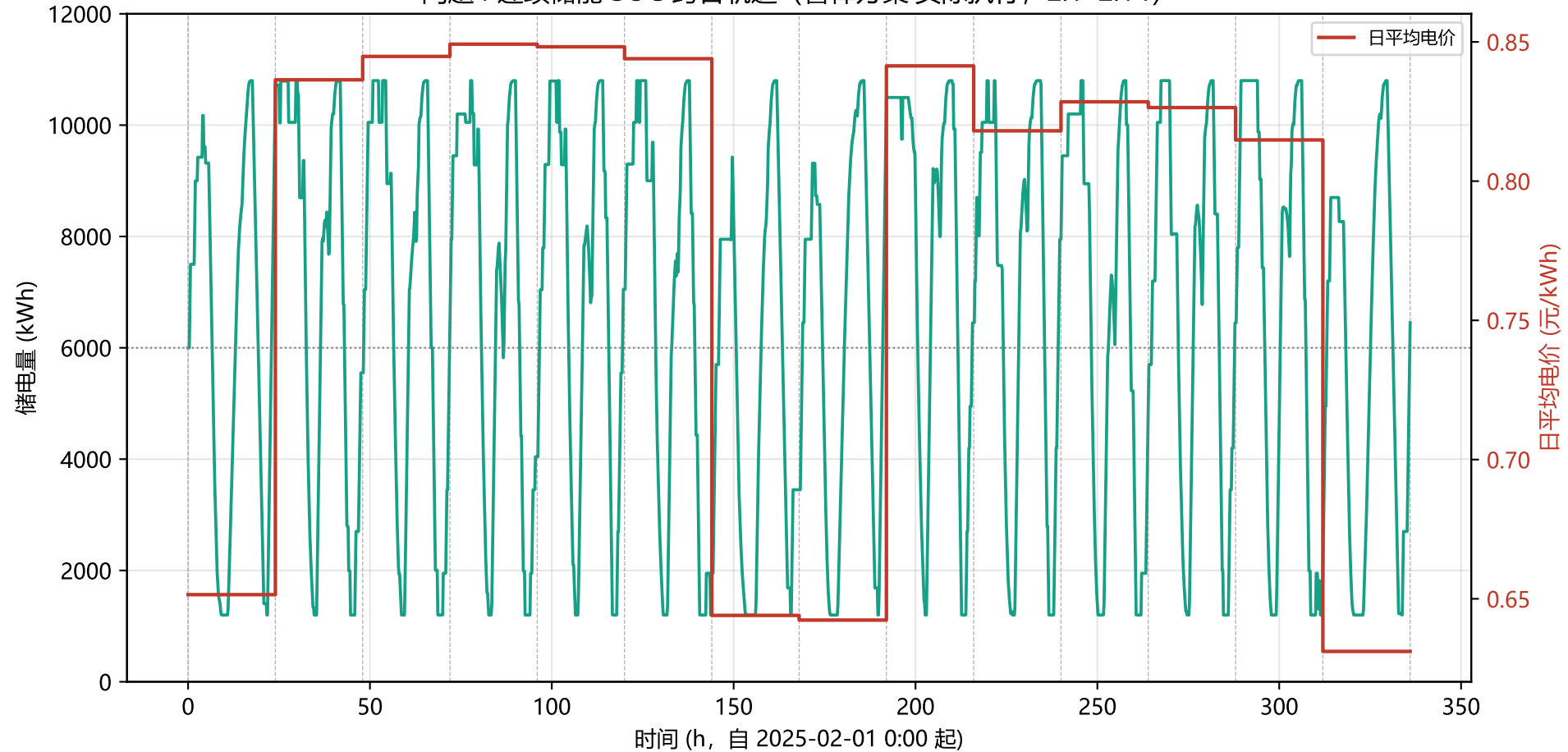
问题4 连续储能 SOC 跨日轨迹 (鲁棒方案·实际执行, 2.1-2.14)
