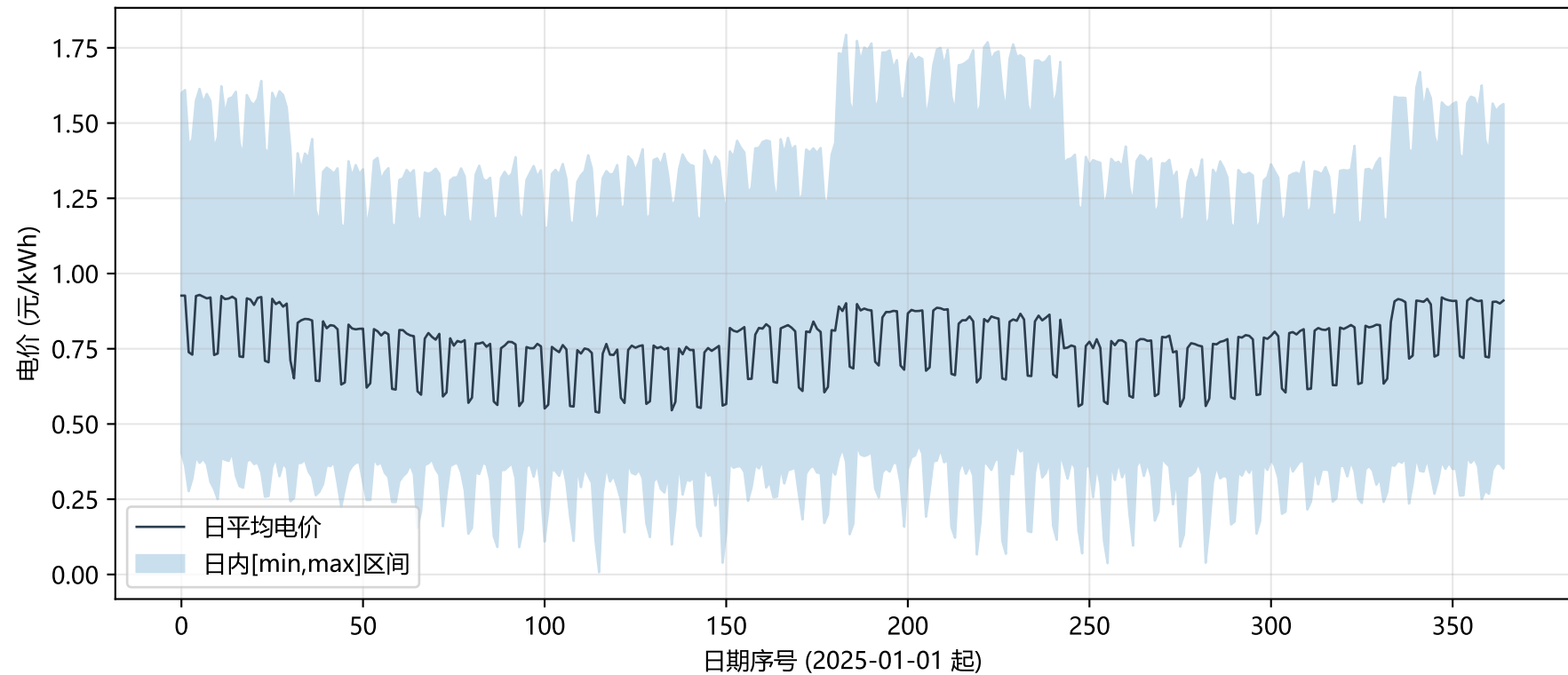
问题4 附件4 全年波动电价
