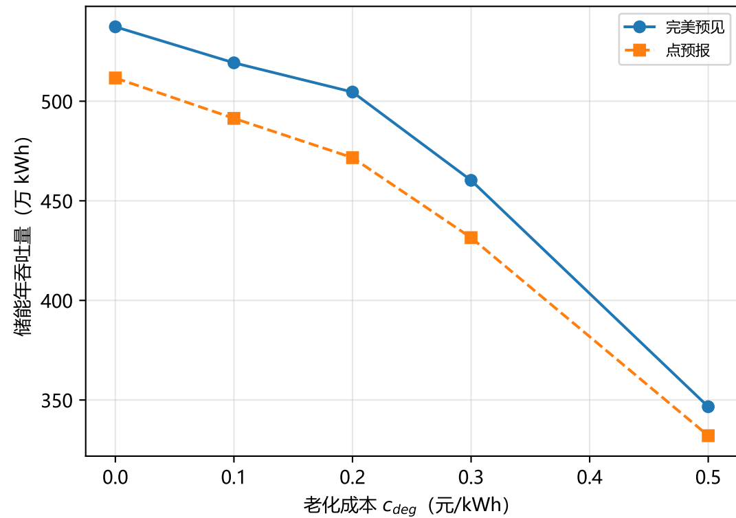
老化成本抑制储能吞吐
