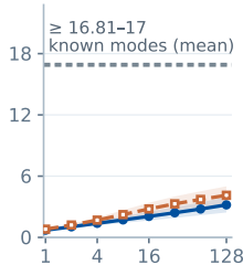
PantryPlan
