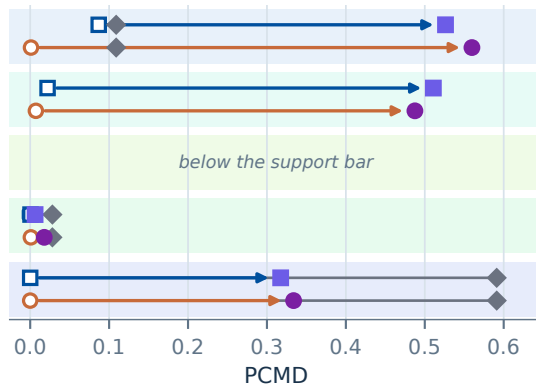
D Falcon3-1B · PCMD
