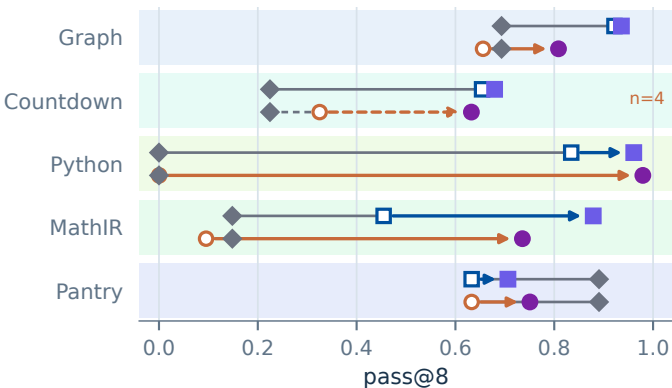
C Falcon3-1B · pass@8
