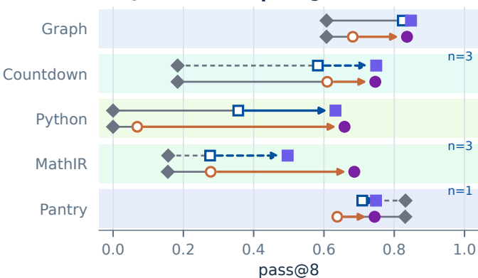
E Qwen2.5-3B · pass@8
