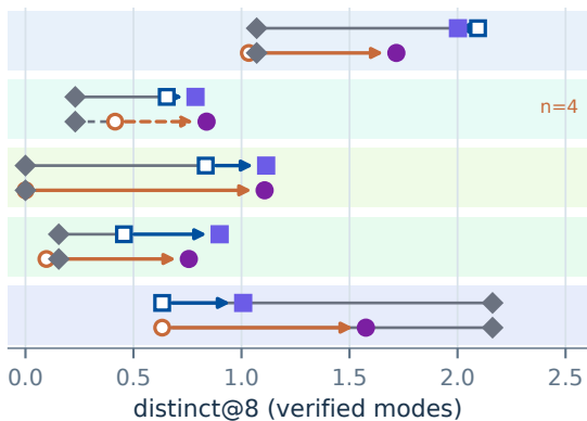
D Falcon3-1B · distinct@8
