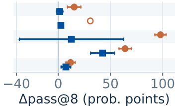
Falcon3-1B
