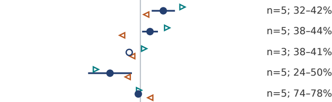
Falcon3-1B
