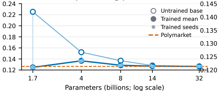
Qwen3 checkpoints (log parameter scale)
