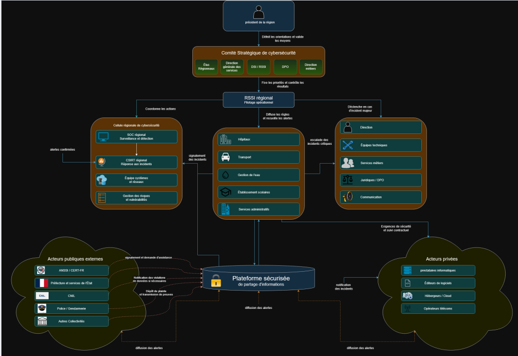
Schéma – gouvernance locale de la cybersécurité (pilotage, contrôle, coordination et partage d'informations)
