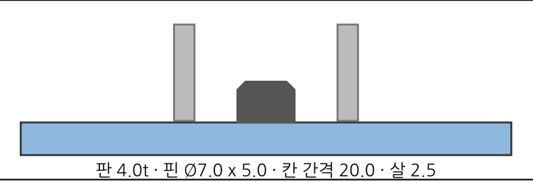
단면 (핀이 격자 칸에 들어간 모습, 위아래 반전)
