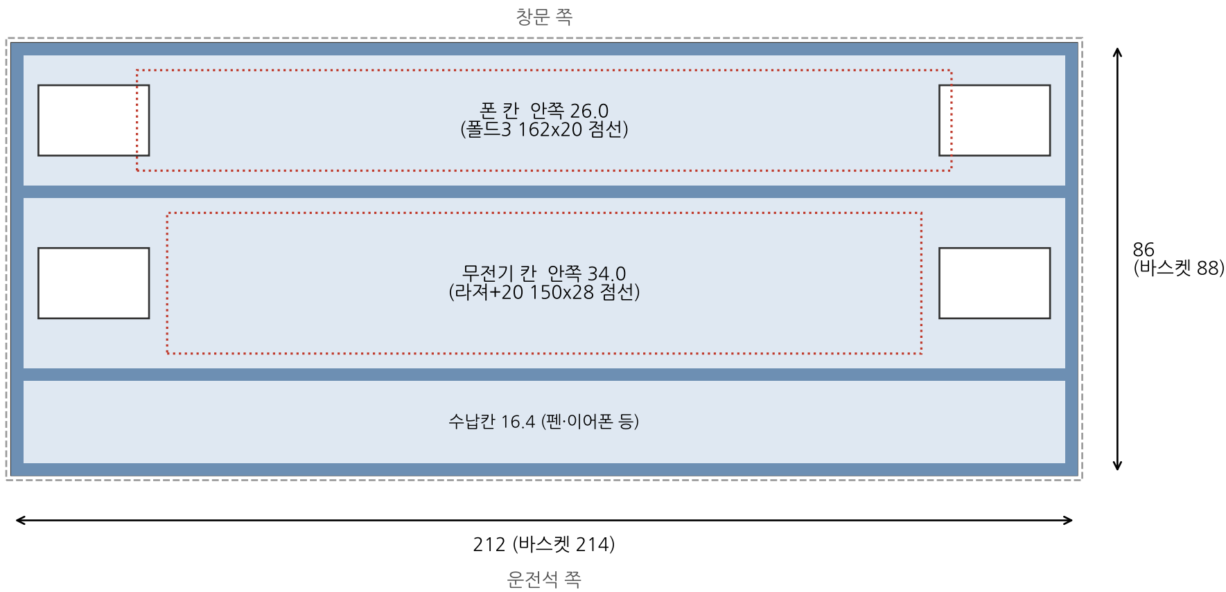
평면도 (흰 사각형 = 케이블 구멍)
