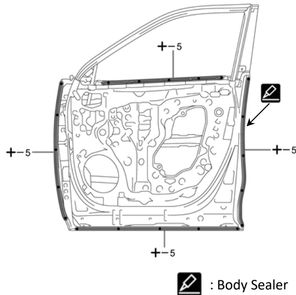
Fig. 1 Body Sealer + Spot MIG Weld
