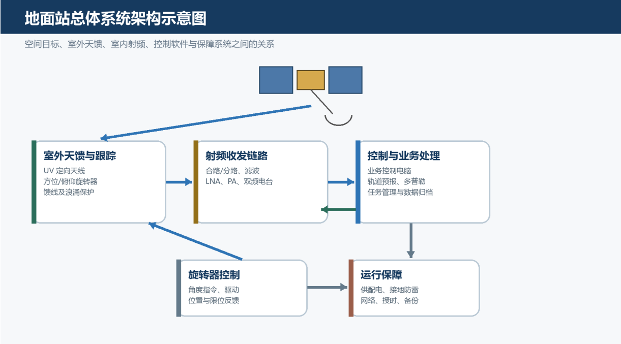
图 2-3 地面站总体系统架构示意图
