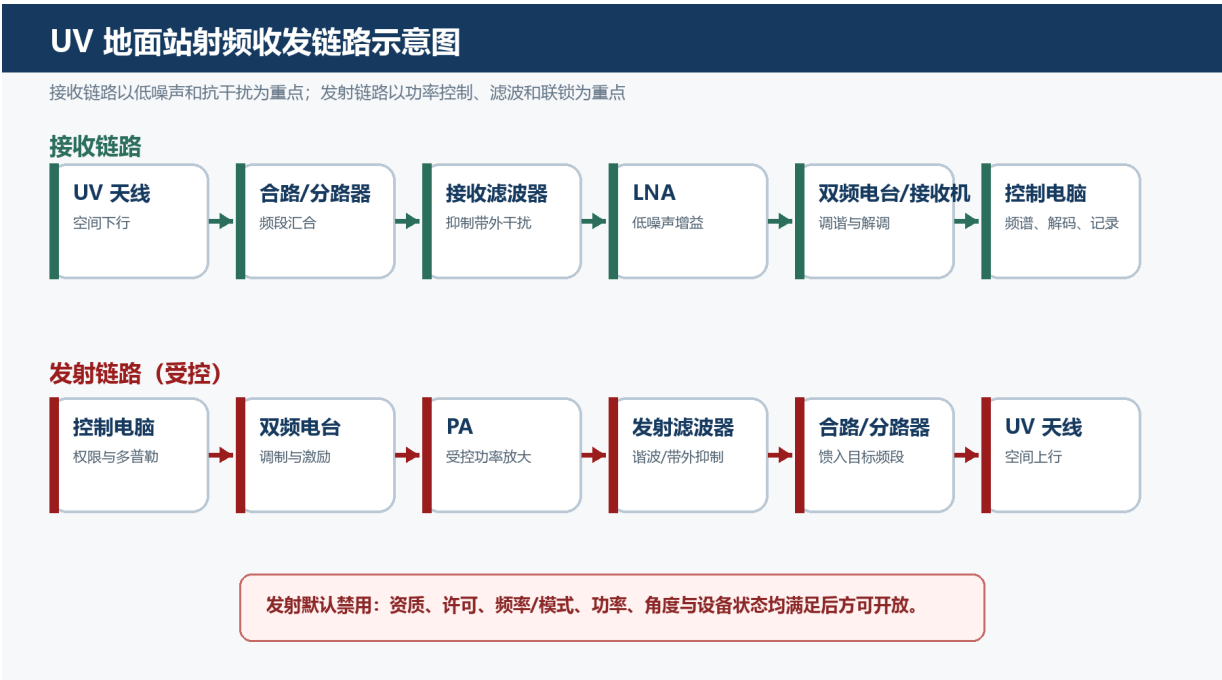
图 2-4 射频接收与受控发射链路示意图
