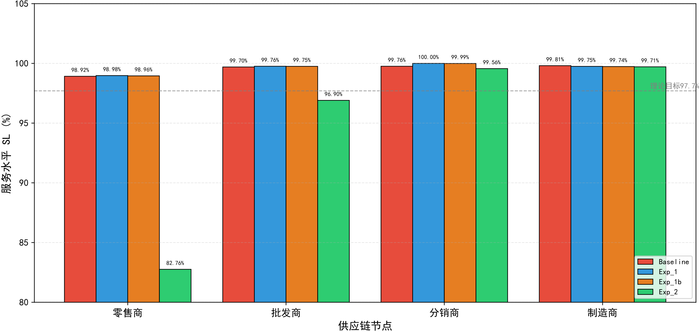
四组实验服务水平对比（20000周期）
