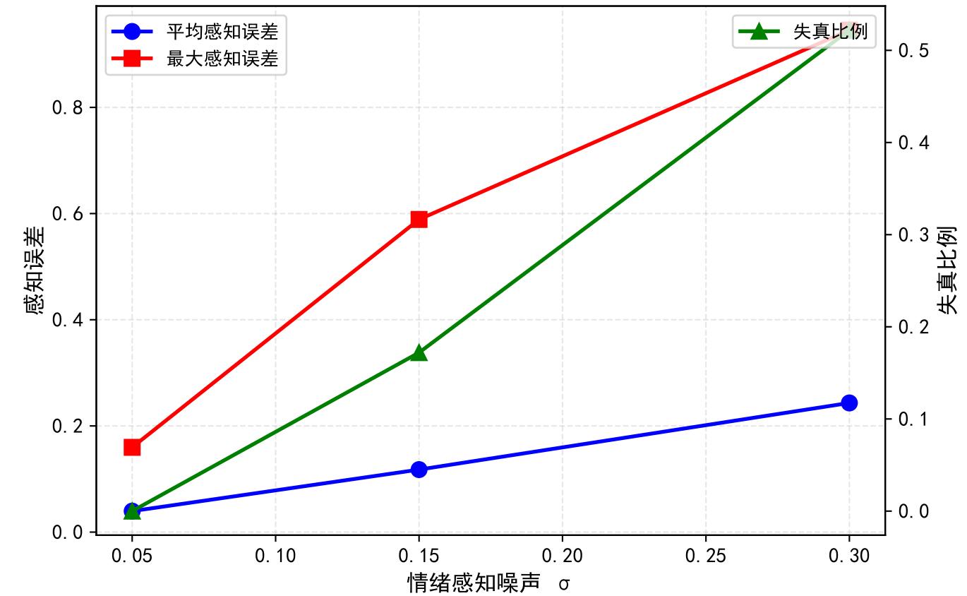
(c) 情绪感知噪声 \sigma 敏感性
