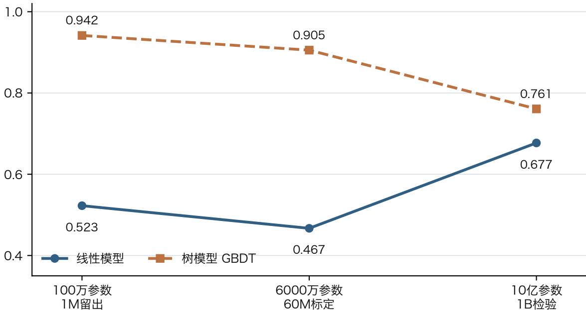
预测与实测配比优劣顺序的一致性 Spearman 相关系数 (越高越一致)
