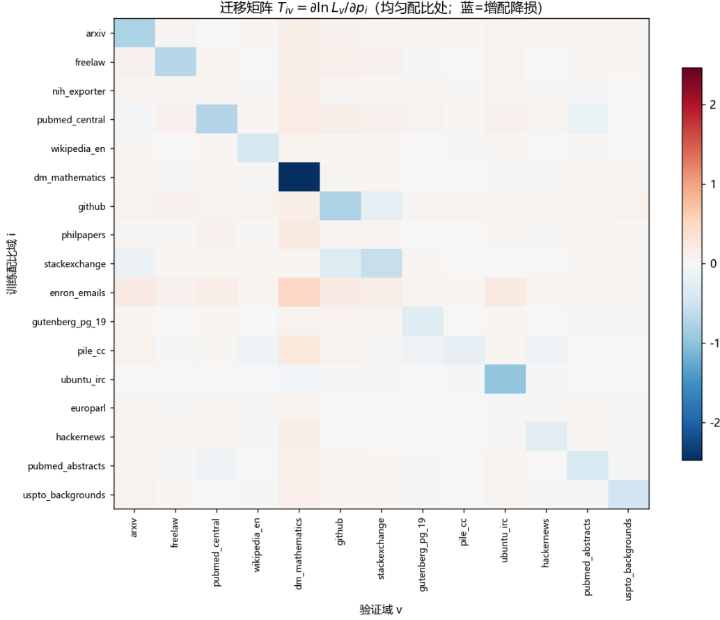
图 10 17 × 13 迁移矩阵：各验证域对训练域份额的局部敏感度
