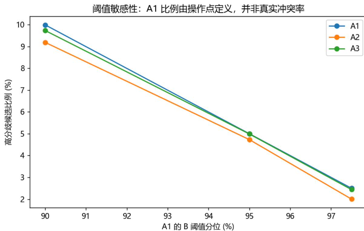
图 4 候选比例对筛查阈值的敏感性
