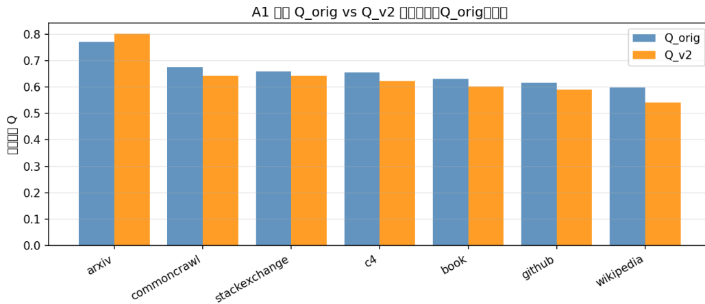
图7 折扣对照分与主分的域级中位数对照
