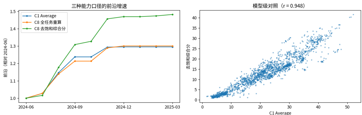
图 19 去饱和分与 C1 Average 的历史窗口比较
