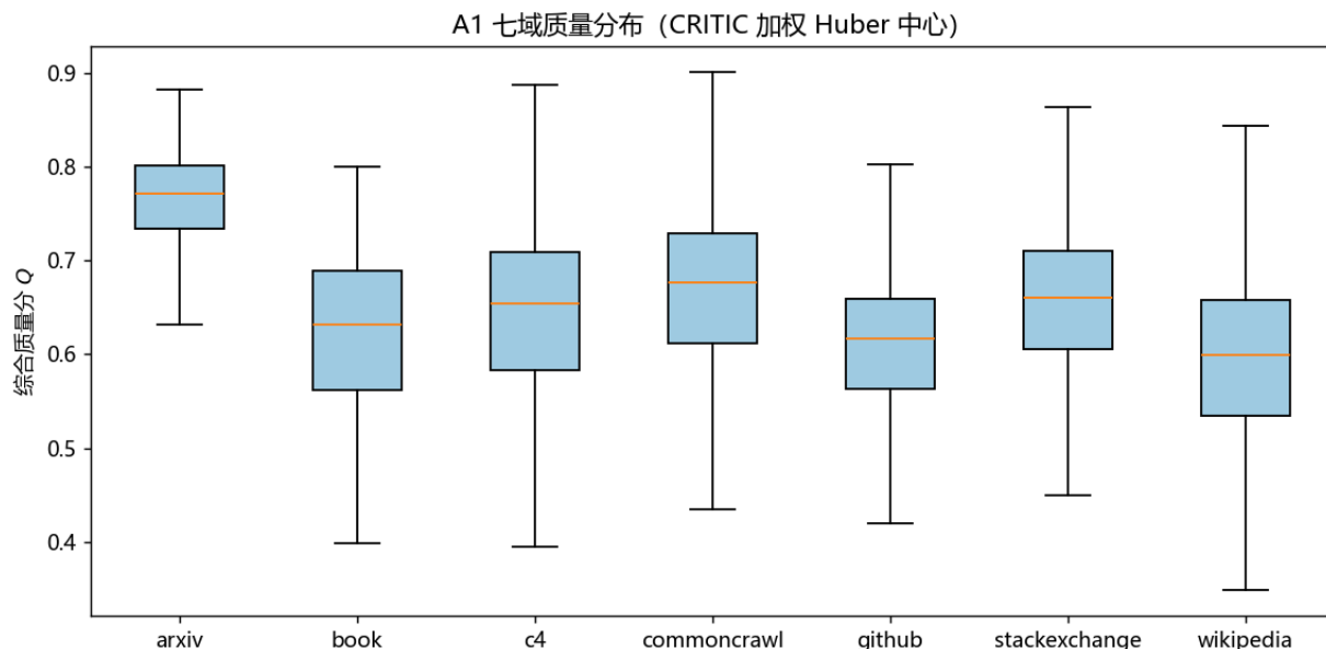
图 1 A1 七域的 CRITIC 加权 Huber 主分分布
