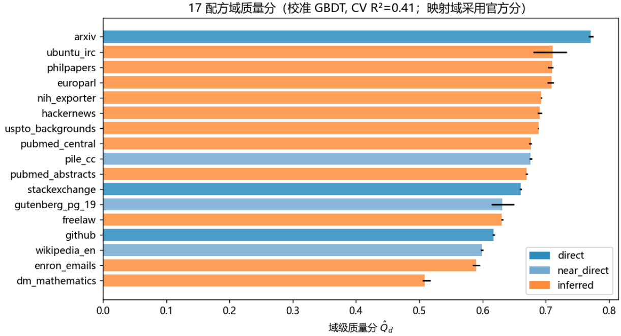
图 9 17 个配比域的质量分与条件区间
