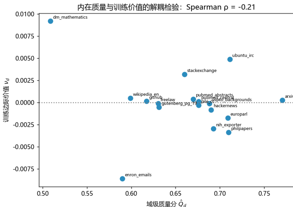
图 14 17 域质量分与训练边际价值的散点关系
