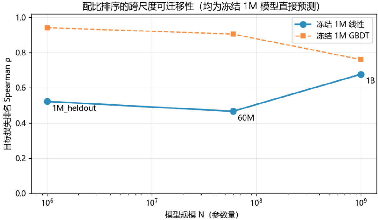
图 11 冻结 1M 配比模型在 1M 留出、60M 与 1B 上的排序保持度
