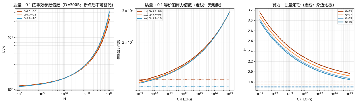
图 16 等效参数倍数、等价算力倍数随预算变化与算力—质量前沿
