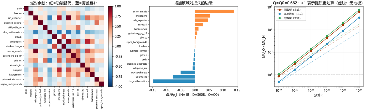
图 17 域对余弦热力图、份额边际与 MU_Q/MU_N 随预算变化
