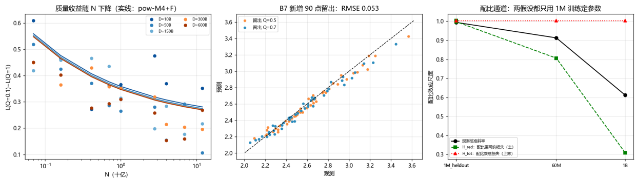
图 15 质量项候选比较与 B7 新增 90 点的留出表现
