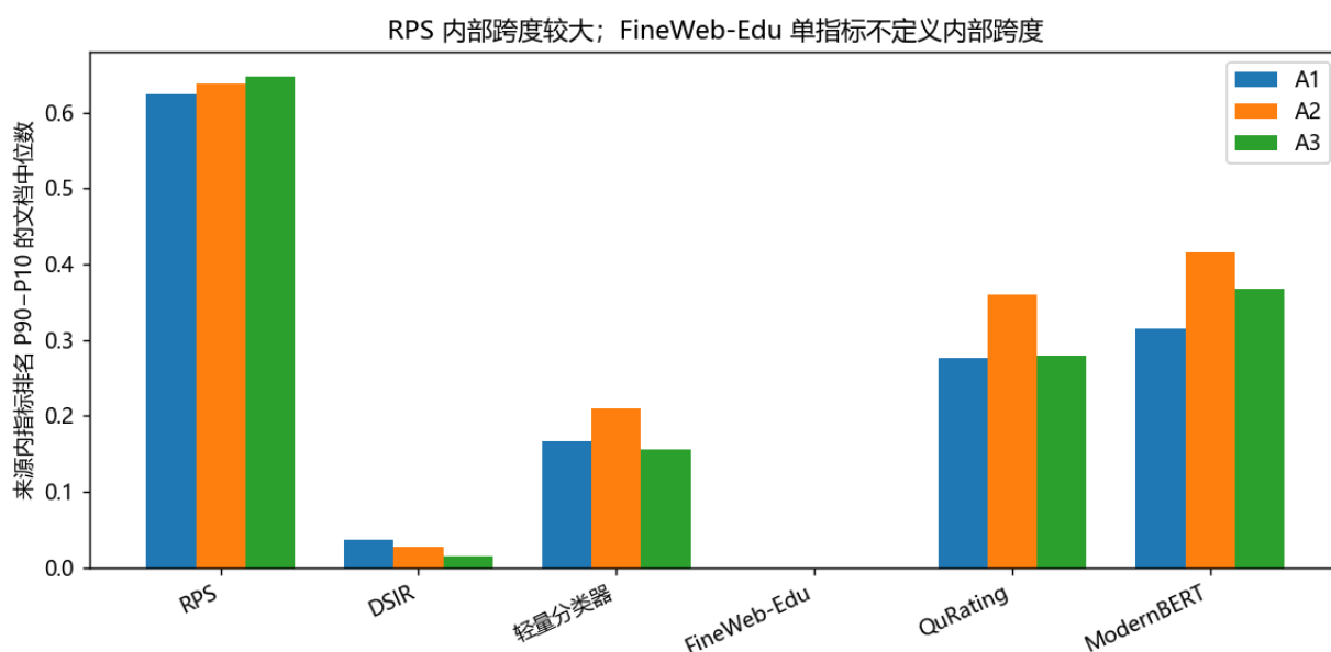
图 2 A1 六来源内部跨度与一致性对照
