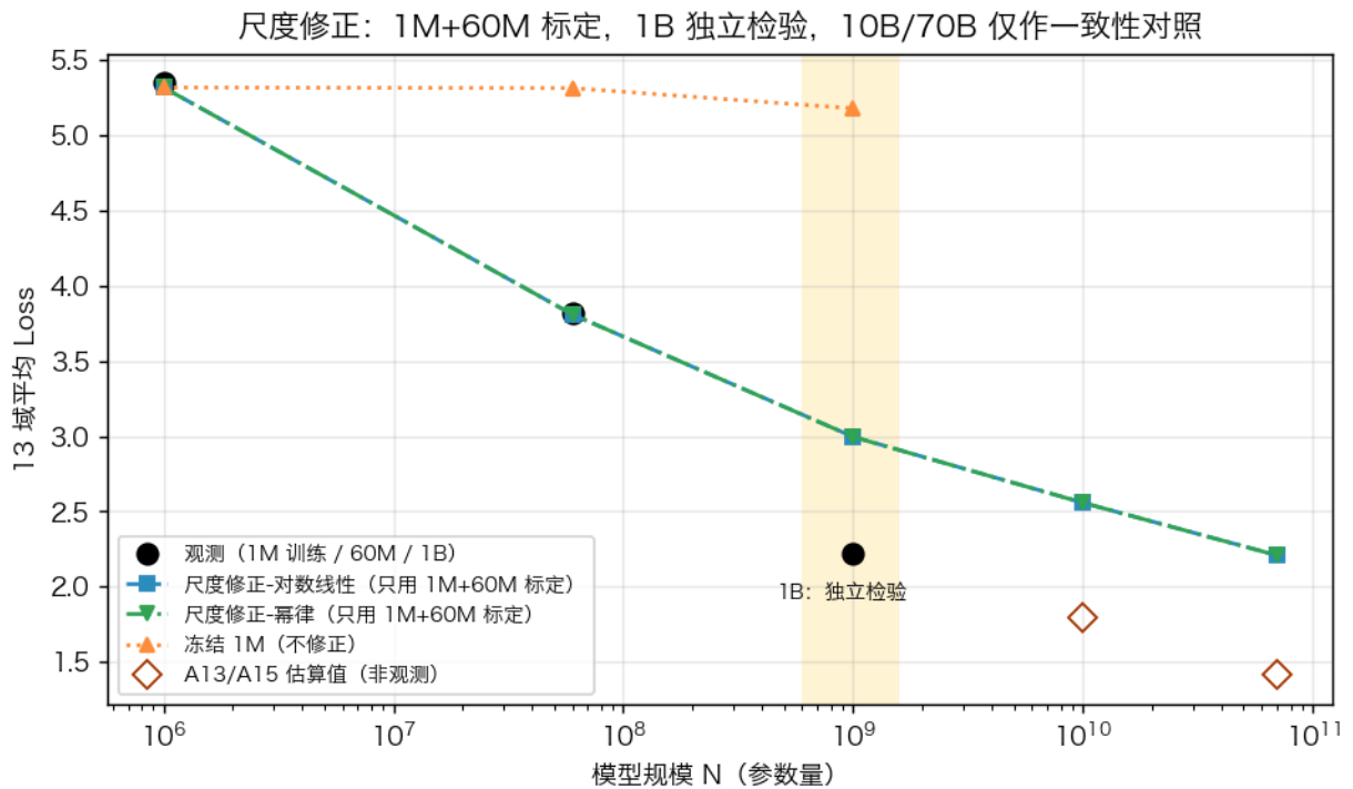
图 12 尺度修正前后的绝对损失对照 (1M + 60M 标定, 1B 独立检验)
