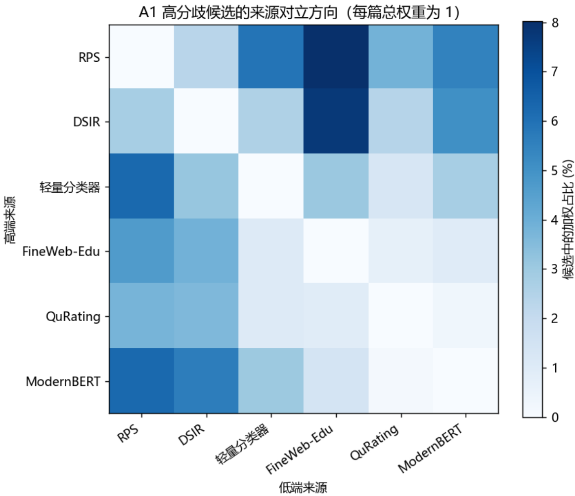
图 3 六来源对立方向的加权份额
