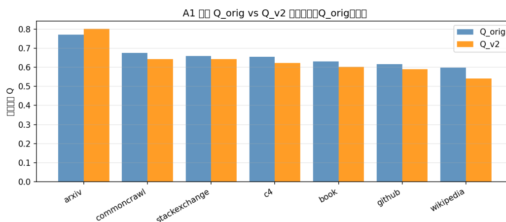
图 22 来源一致性加权实验分与主分的域级中位数对照
