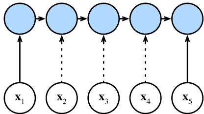
循环神经网络
