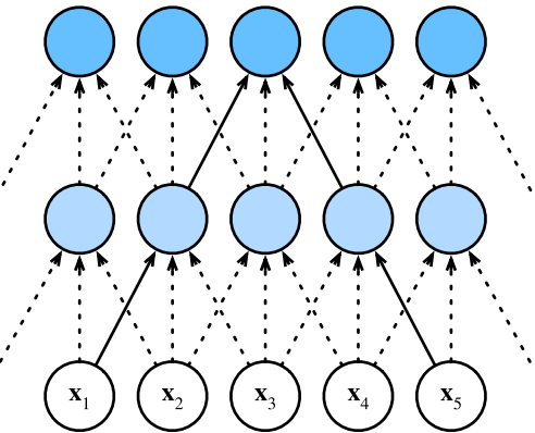
卷积神经网络
