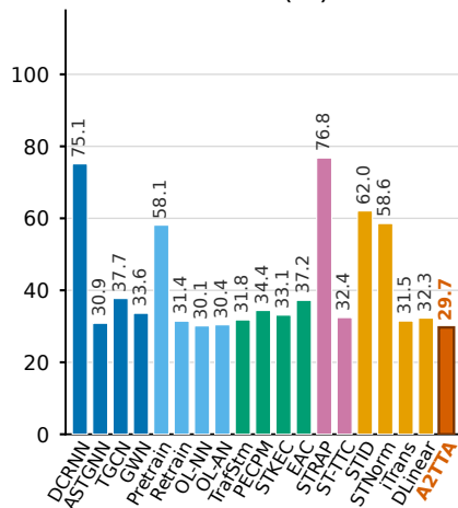
MAPE (%)
