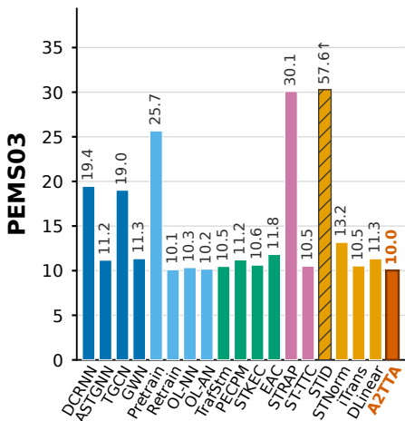
MAE
