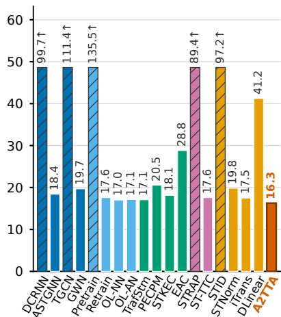
PEMS04
