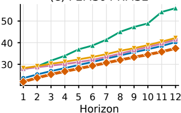
(h) PEMS07 RMSE
