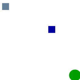
图 1.1 画一些点
