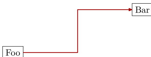
图 3.5 foo → bar
