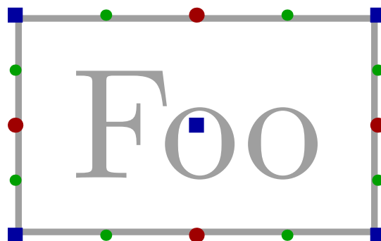
图 3.4 锚点示例
