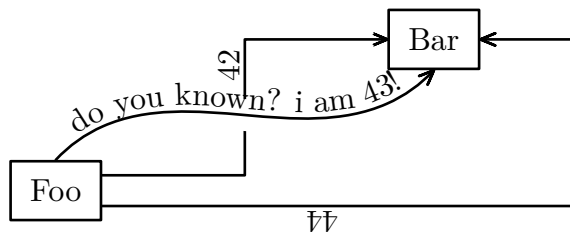
图 13.2 话痨 NPC
