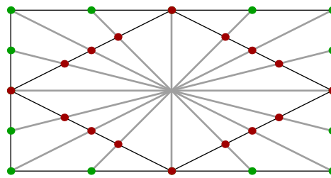
图 6.1 锚点散射
