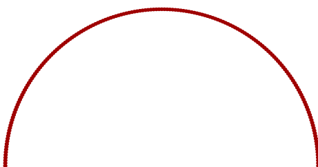
图 1.6 半圆轨迹
