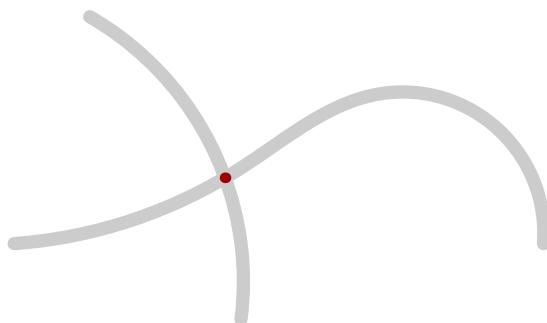
图 5.1 路径求交
