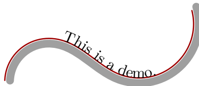
图 7.9 路径偏置
