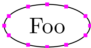
图 6.2 椭圆文本框
