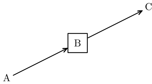
图 12.8 节点直连
