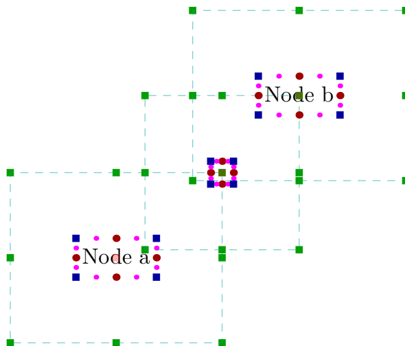
图 11.2 空节点示例
