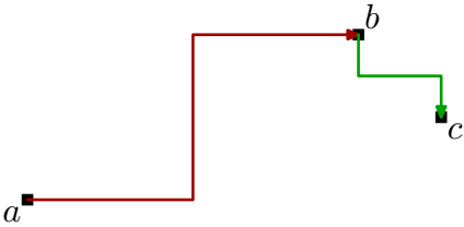
图 2.4 xyxto 与 yxyto 构造的路径
