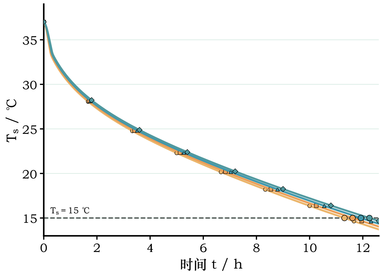
(b) 皮肤温度与 15 ^\circ\text{C} 阈值
