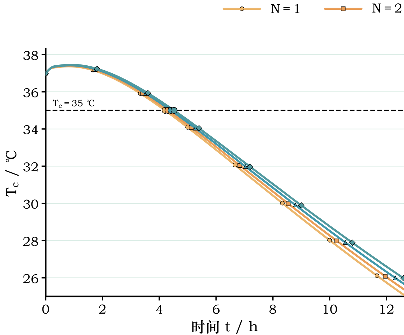
(a) 核心温度与 35 ^\circ\text{C} 阈值
