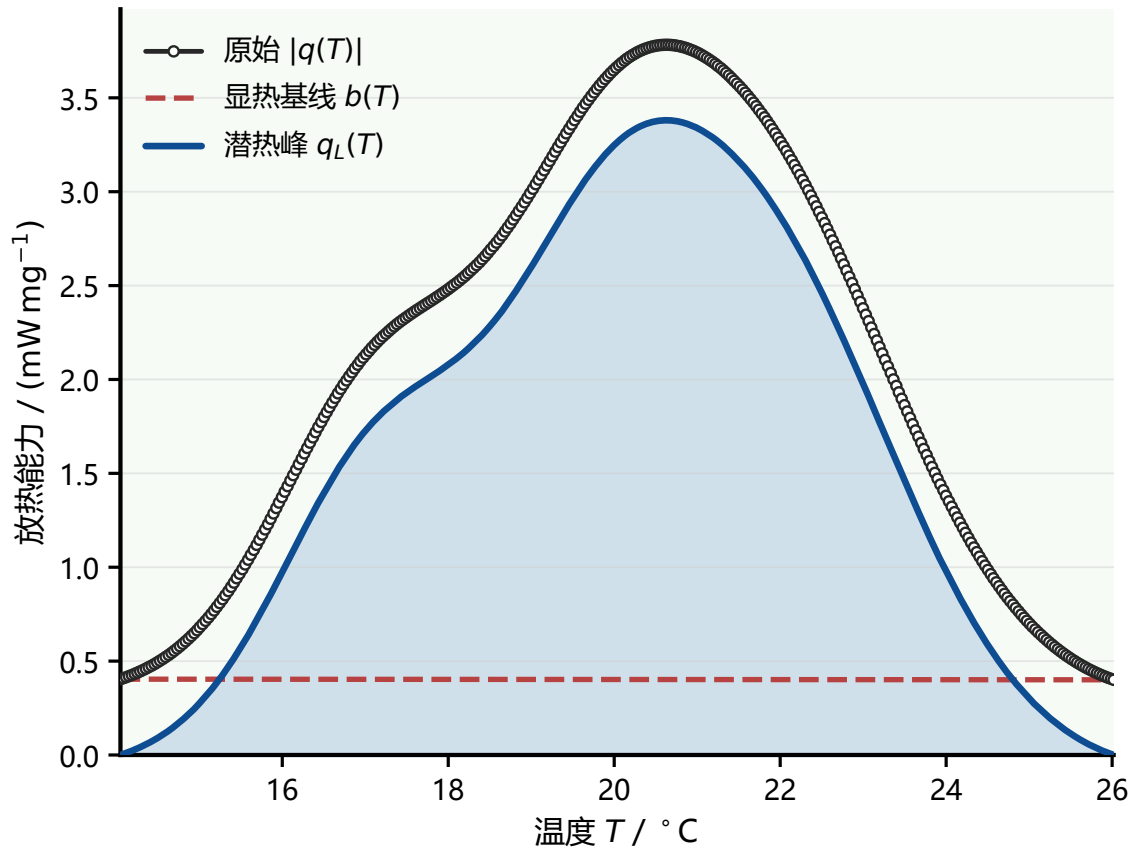
(a) DSC 基线分离与潜热峰
