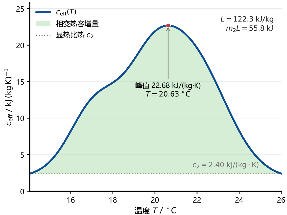
(b) PCM 表观比热
