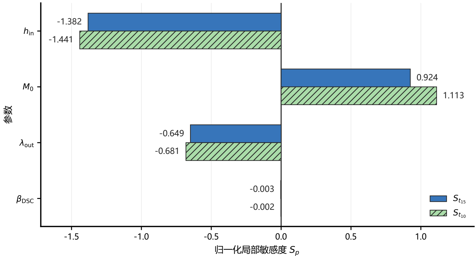
阈值时间的归一化局部敏感度
