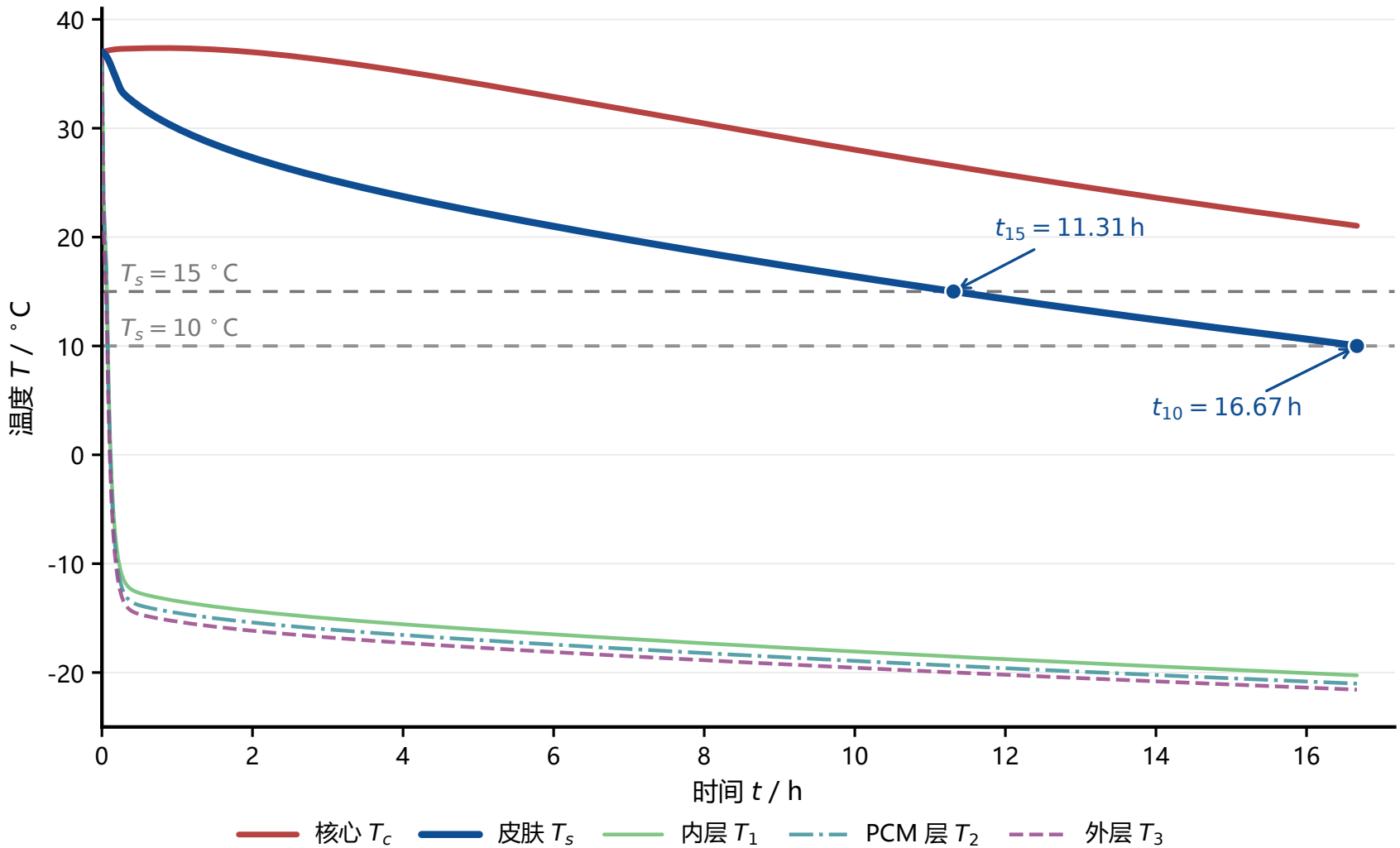
极寒环境下人体—防护服各节点温度响应
