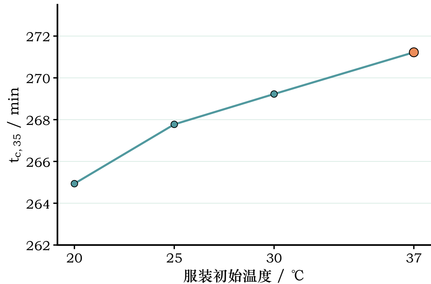
(b) 服装初始温度影响
