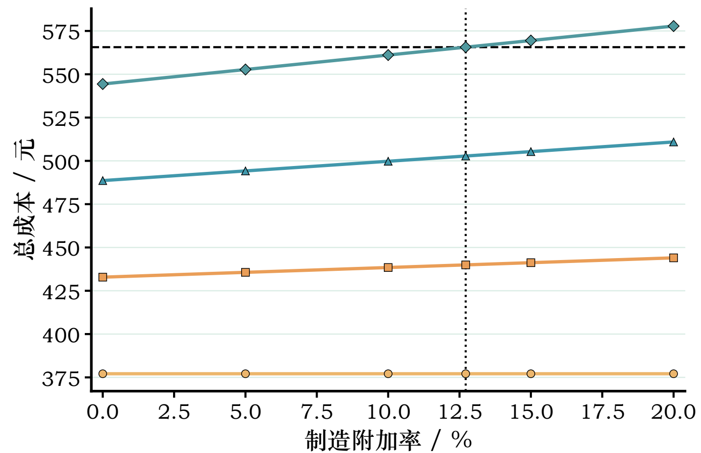
(d) 制造附加率下的总成本
