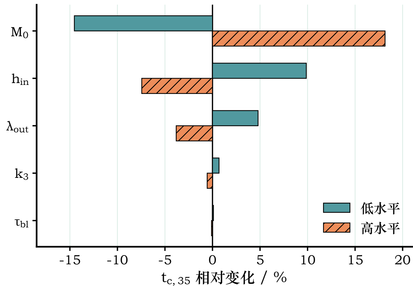
(a) 热学参数单因素敏感性
