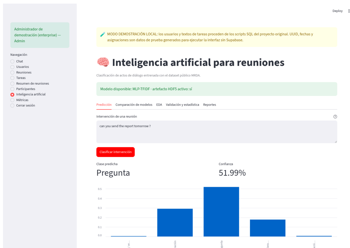
Figura F2. Predicción real consumiendo best_model.h5.
