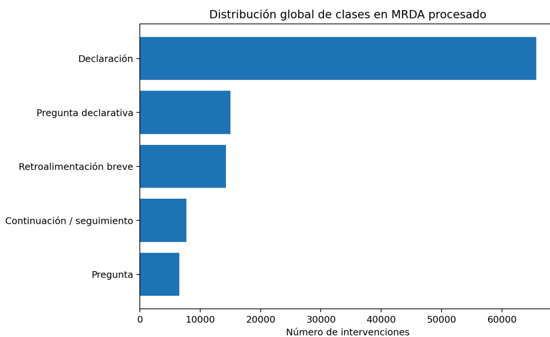
Figura 1. Distribución global de las cinco clases.
