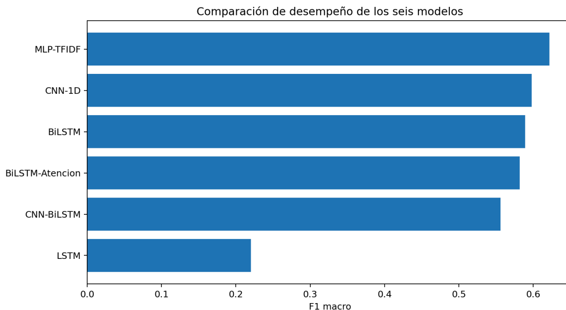
Figura 6. Comparación de F1 macro de los seis modelos.
