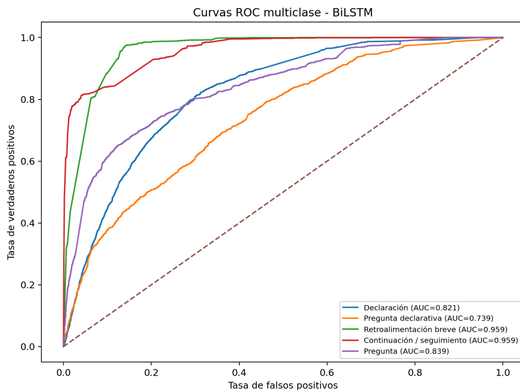
Figura B6. Curva ROC BiLSTM.
