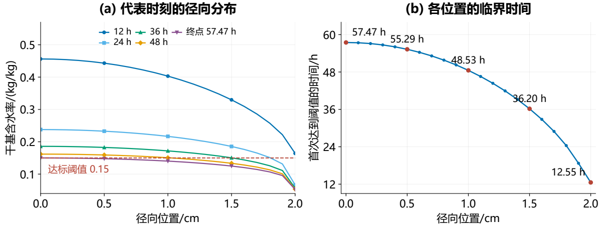
图 8 代表时刻的径向含水率分布及各位置首次达到阈值的时间
