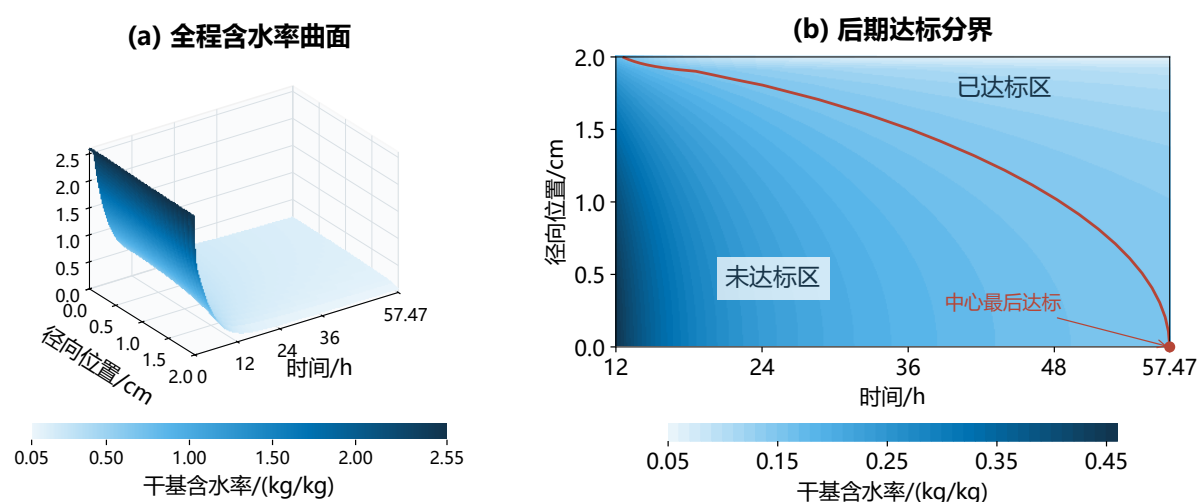
图 7 含水率时空分布及后期达标分界；红线为 C = 0.15 \text{ kg/kg} 等值线
