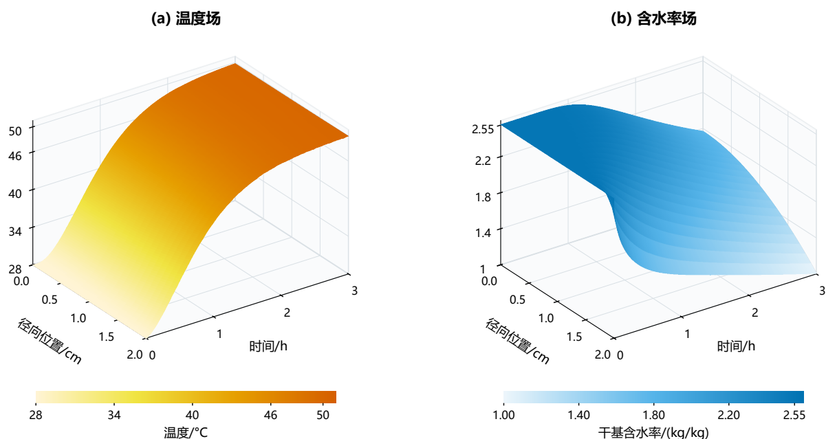
图 5 问题二温度场与干基含水率场的时空演化曲面。横轴为时间，纵轴为径向位置，时间范围为 0–3 h，径向范围为 0–2 cm。
