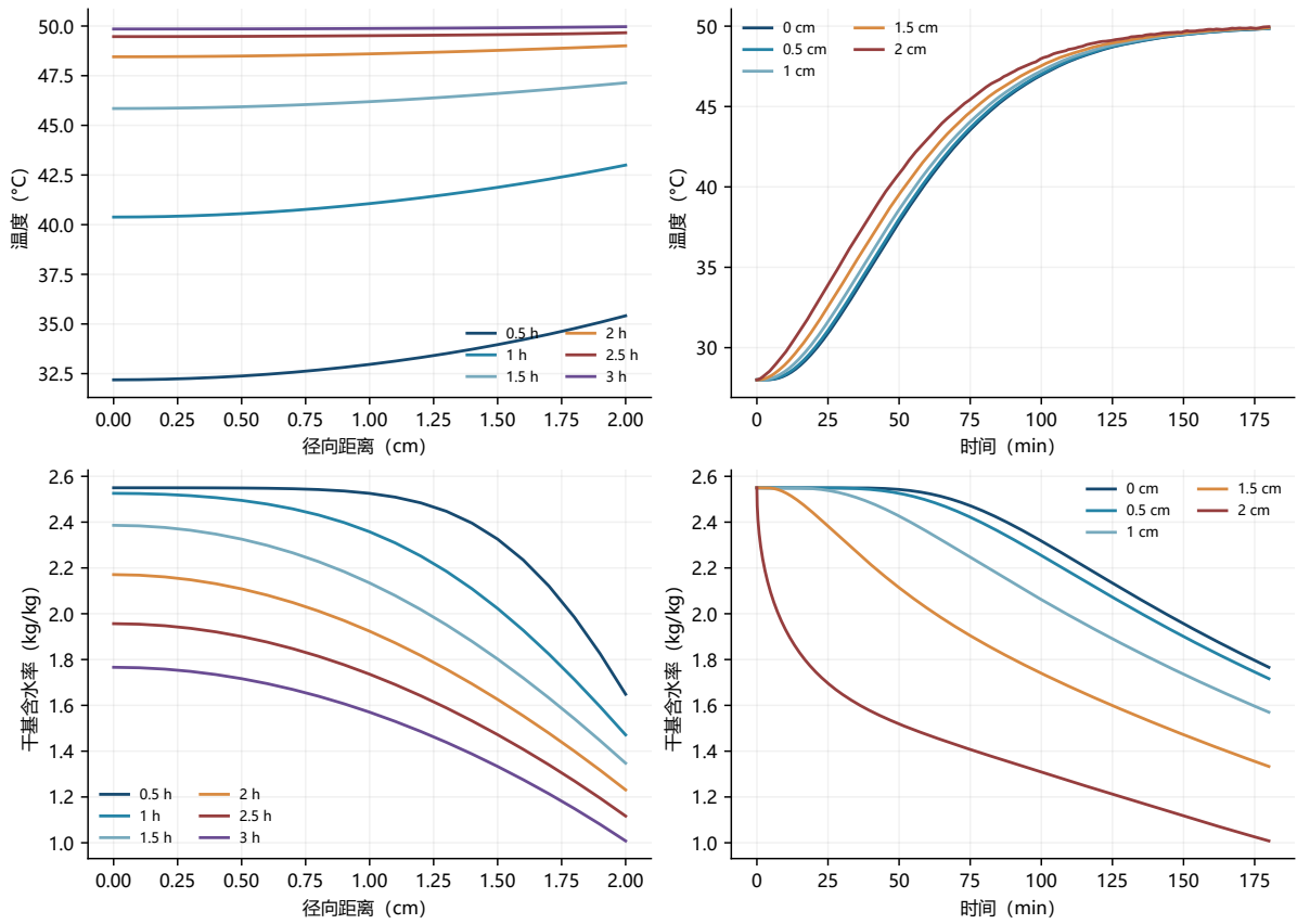
图 4 问题二温度与干基含水率的径向剖面及时间演化。左列为 0.5、1、1.5、2、2.5、3 h 六个时刻的径向剖面，右列为 0、0.5、1、1.5、2 cm 五个位置的时间曲线。
