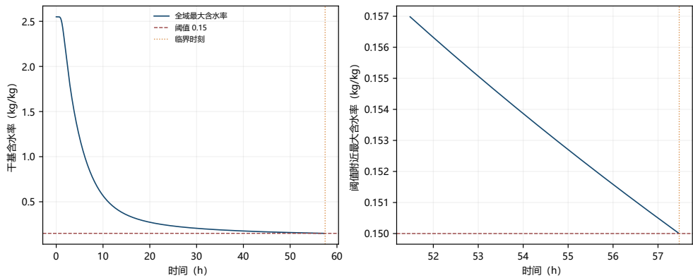
图 6 最大含水率的变化及烘干终点
