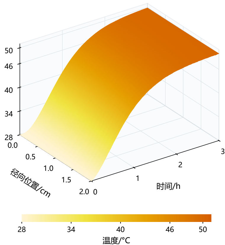
(a) 温度场
