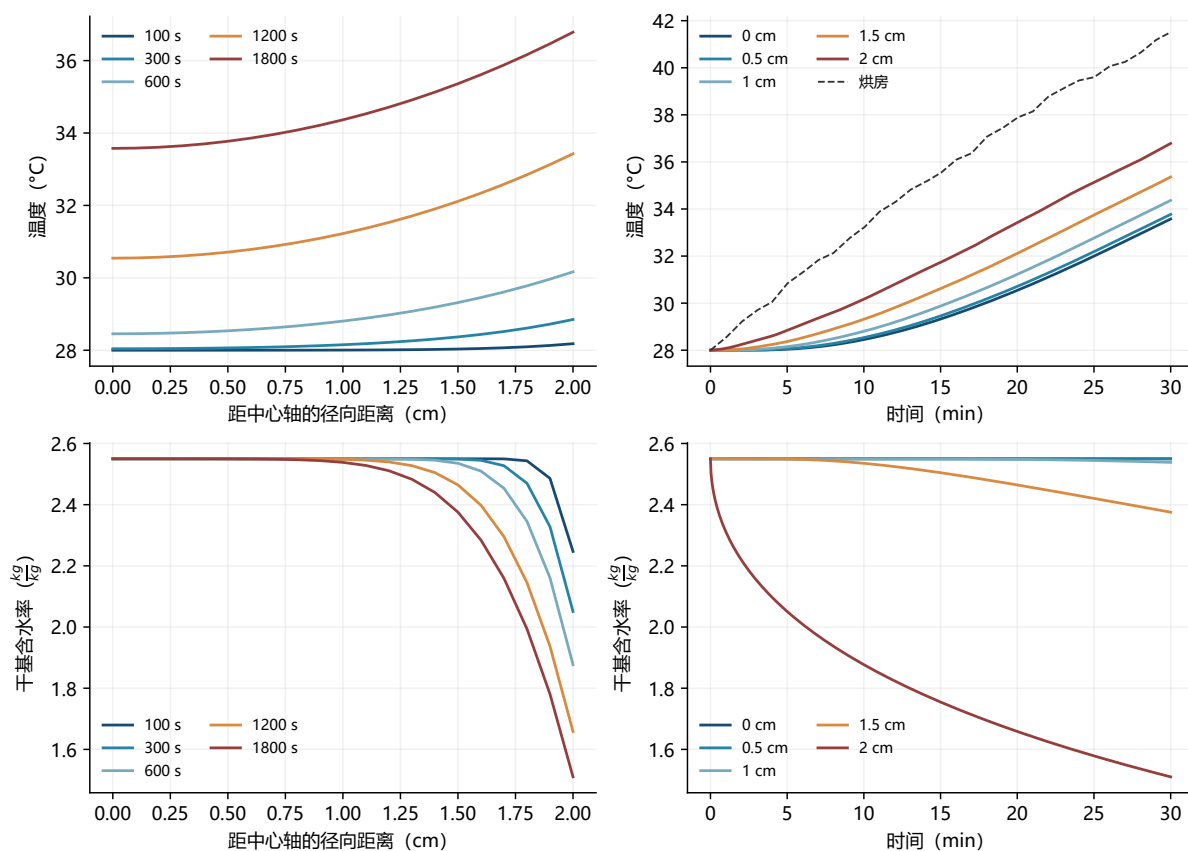
图 3 预热阶段温度与含水率的径向分布及时间变化
