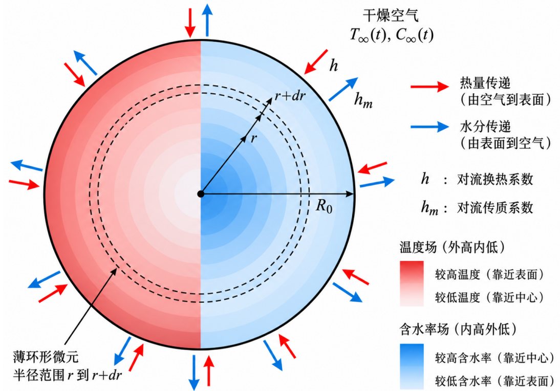
图 2 圆柱药材的径向传递及薄壳微元
