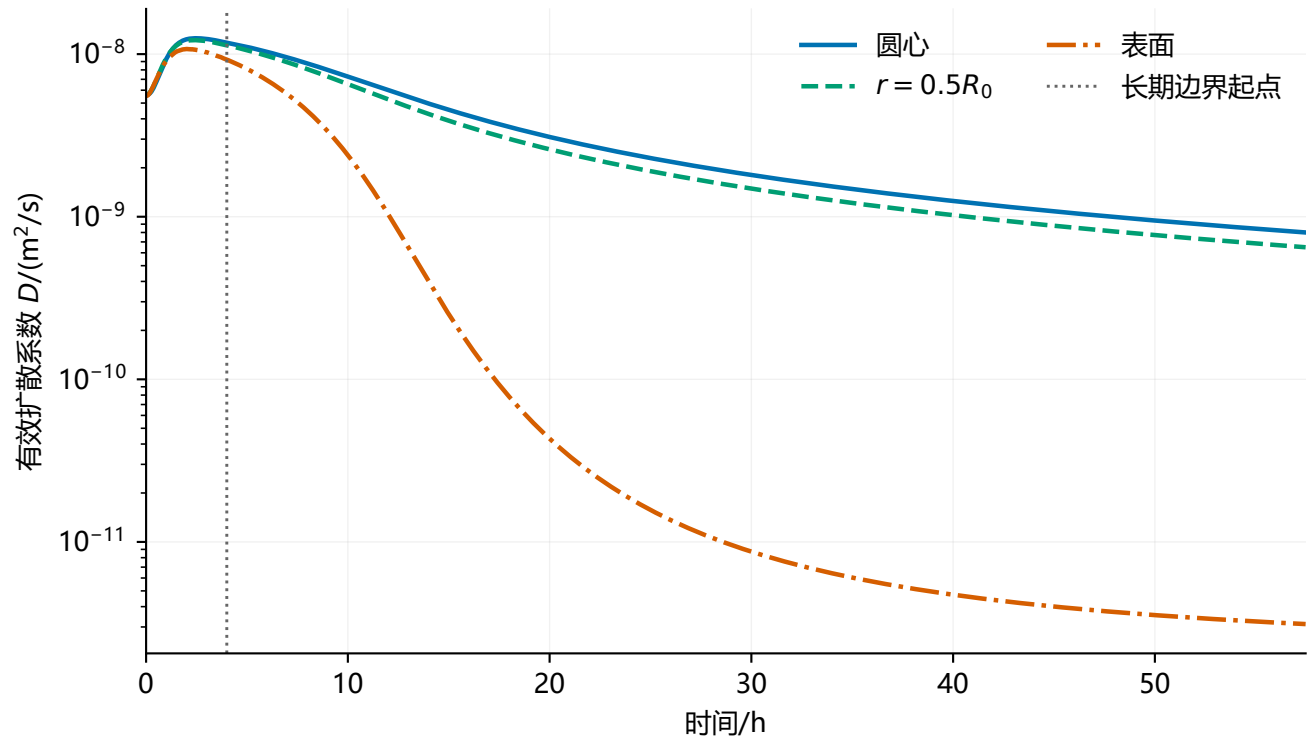
不同径向位置的有效扩散系数
