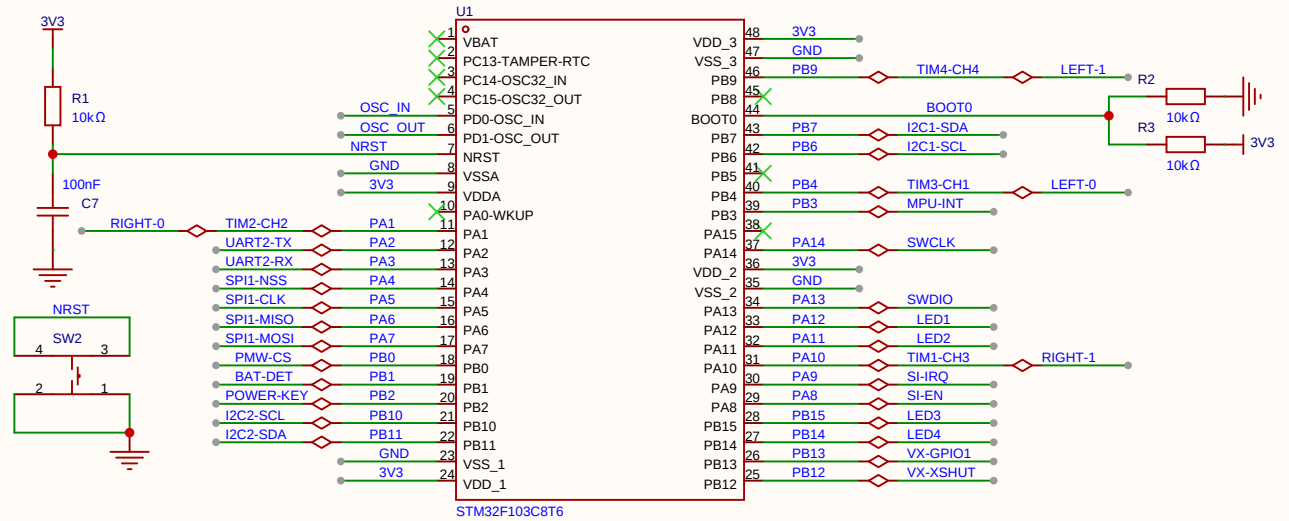
飞控主控STM32
