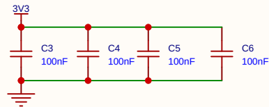
MCU滤波
