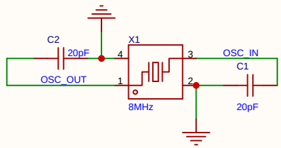
晶振
