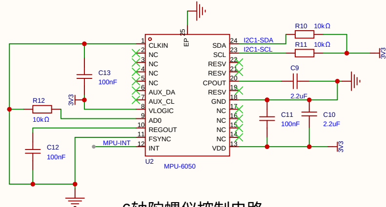
6轴陀螺仪控制电路
