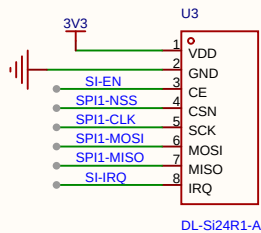
2.4G收发模块
